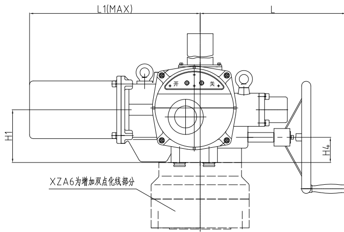
XZA3-6基本型外形尺寸
